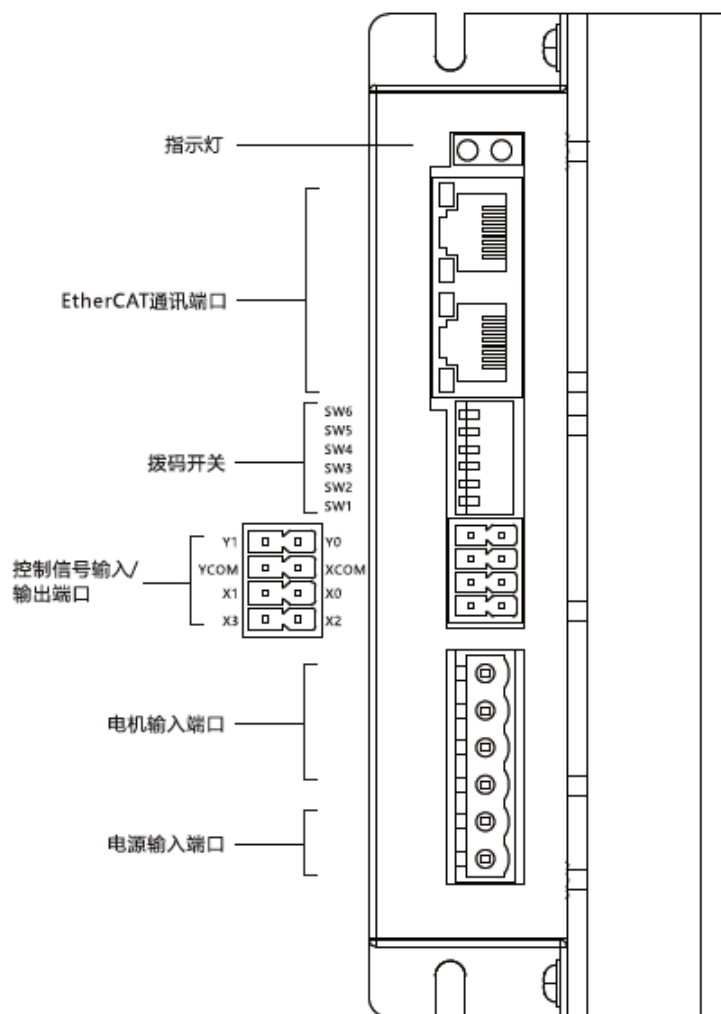
驱动器侧面端口示意图
